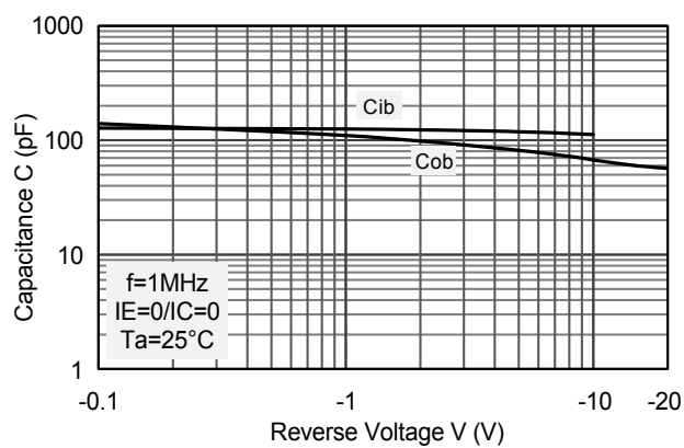
Fig8.Cob/Cib——VCB/VEB
