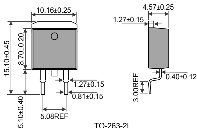
TO-263-2L Unit:mm
